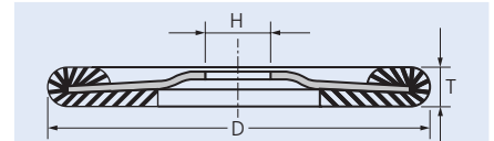
Lamelový kotouč, radiální typ PFR (CURVE)
