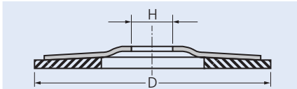
Lamelový kotouče, plochý typ PFF (tvar A)
