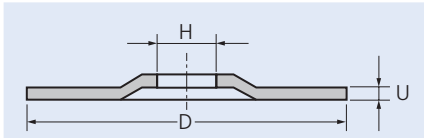
Brusný kotouč E (tvar 27) nebo řezací kotouč, provedení se sníženým středem EH (tvar 42)
