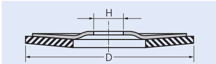
Lamelový kotouče, kuželový typ PFC (tvar B)
