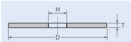
Řezací kotouč, ploché provedení EHT (tvar 41)
